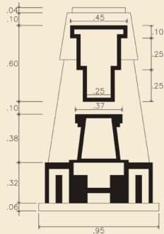
ELEVACIONES ESC 1/10
